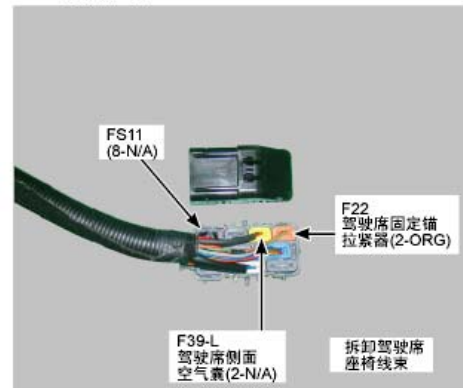
228.驾驶席座椅
